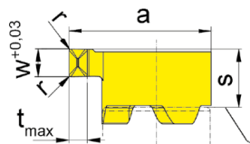
Klemmhalter Stirnseite Toolholder face
