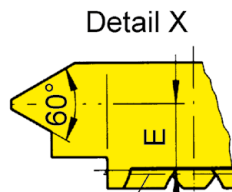
Klemmhalter Stirnseite Toolholder Face
