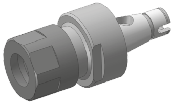
Drehhalter Typ ER11 Turning holder type ER11
